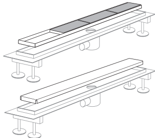
IndorTec® DR-FM Sprchový žlab s roštem pro osazení dlažbou
