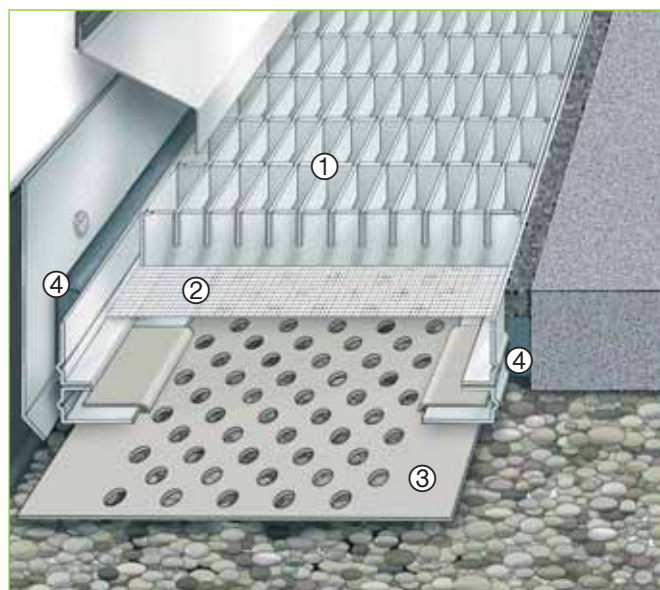
AquaDrain® Vario při aplikaci u balkonových dveří
