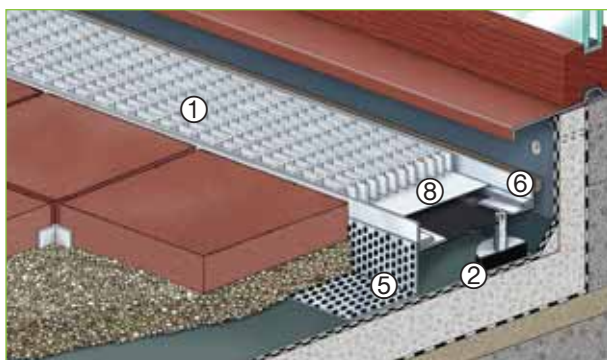
AquaDrain® Flex s pokládkou dlažby bez lepení na podrovnávku ze štěrku /drti
