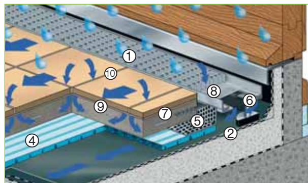
AquaDrain® Flex s pokládkou dlažby na potěrovou vrstvu na AquaDrain® FE+
