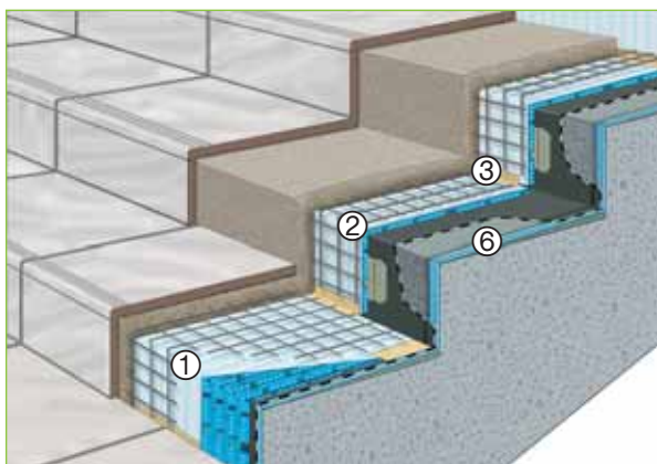
AquaDrain®SD Stufendrainage – Typ 1 s keramickým obkladem
