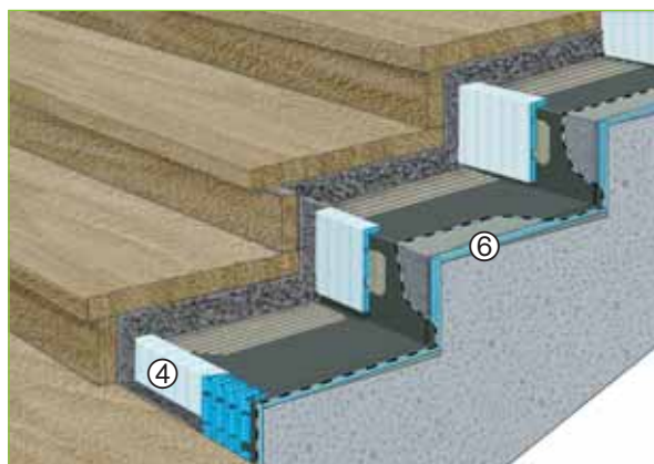
V kombinaci s Watec® 4E v nášlapné části schodu AquaDrain®SD Stufendrainage – Typ 2 v kombinaci na jednozrnné maltě pod přírodním/umělým kamenem.
