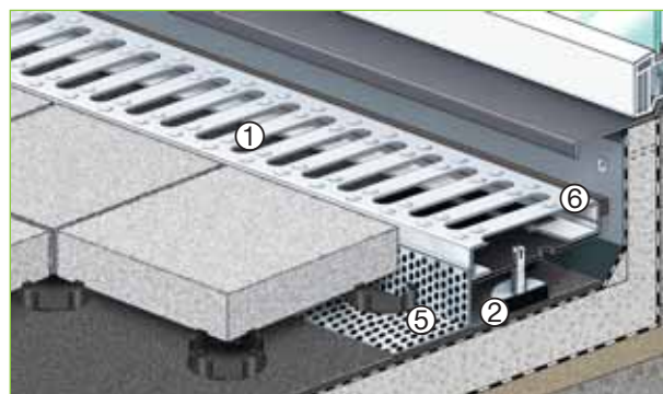
AquaDrain® Flex v kombinaci s terčí
