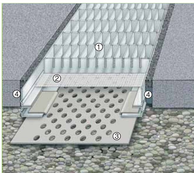
AquaDrain® Vario pro lineární odvodnění
