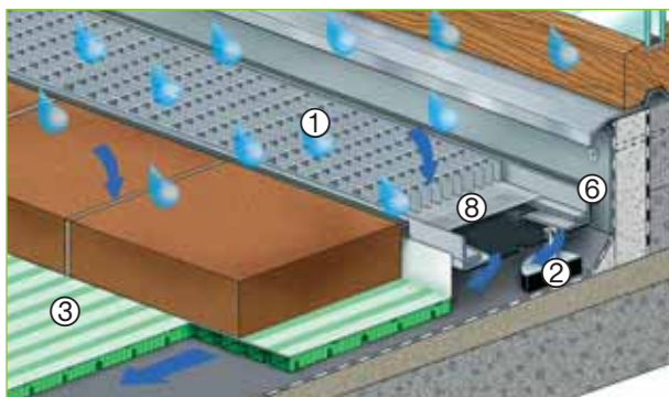
AquaDrain® Flex s přímou pokládkou dlažby bez lepení na AquaDrain® T+
