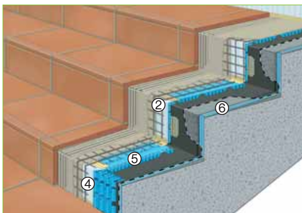
Stufendrainage – Typ 2 v kombinaci s Watec® 4E v nášlapné části schodu
