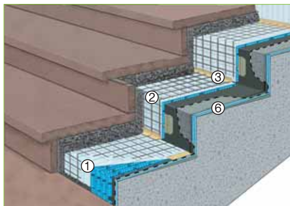
AquaDrain®SD Stufendrainage – Typ 1 s přírodním/umělým kamenem do potěru AquaDrain®SD
