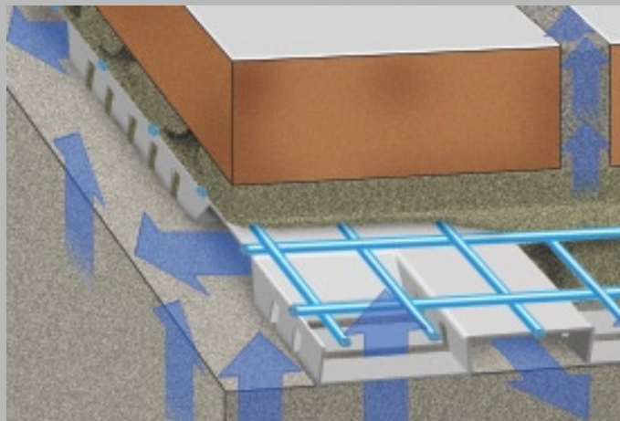
Obrázek 1: Watec 2E odvádí vlhkost kanály v rohoži a současně odvětrává sparami mezi dlažbou.
